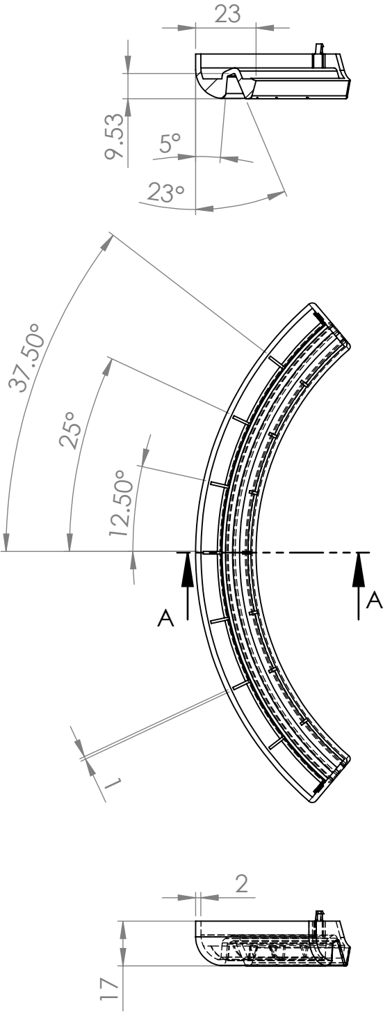
SECTION A-A
